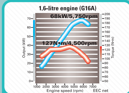
Động cơ trang nhôm 16 van 1.6 lít mạnh mẽ & tiết kiệm nhiên liệu
